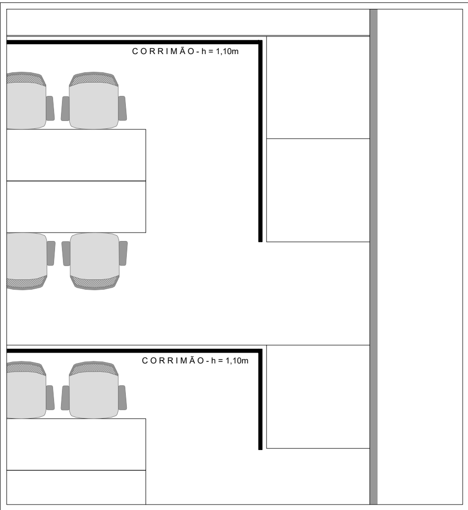
DETALHE - CORRIMÃO
