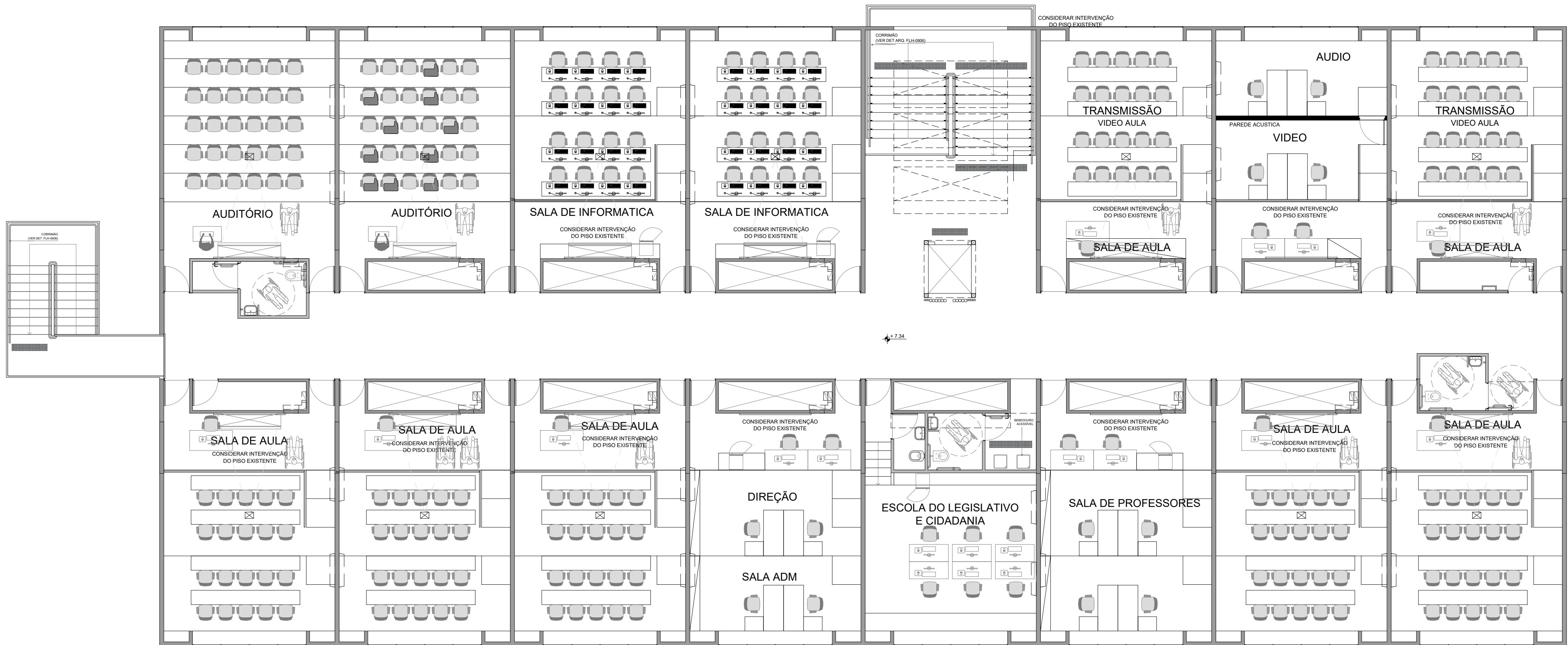
SEGUNDO PAVIMENTO
