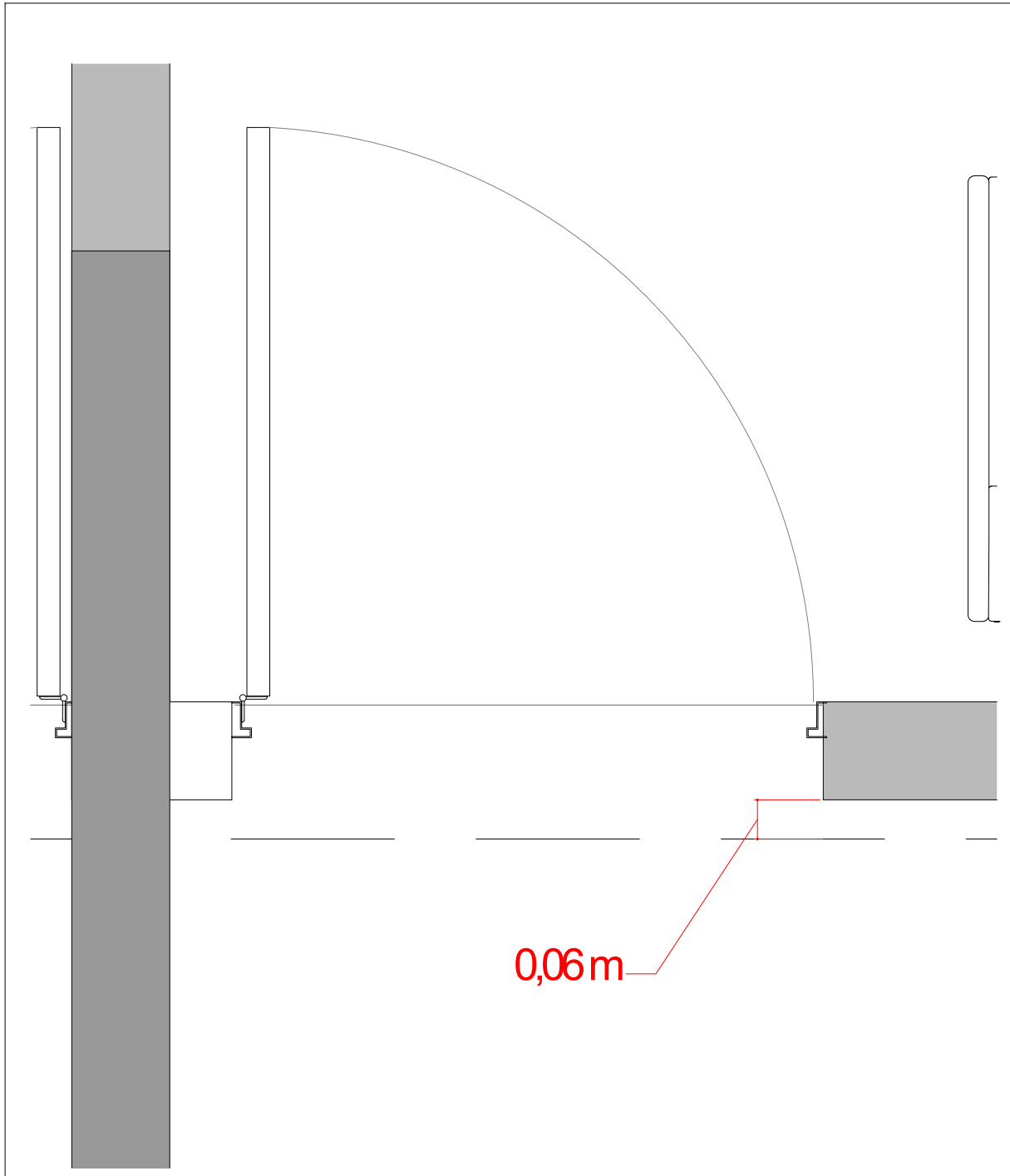
DETALHE - AFASTAMENTO DO CAXILHO
