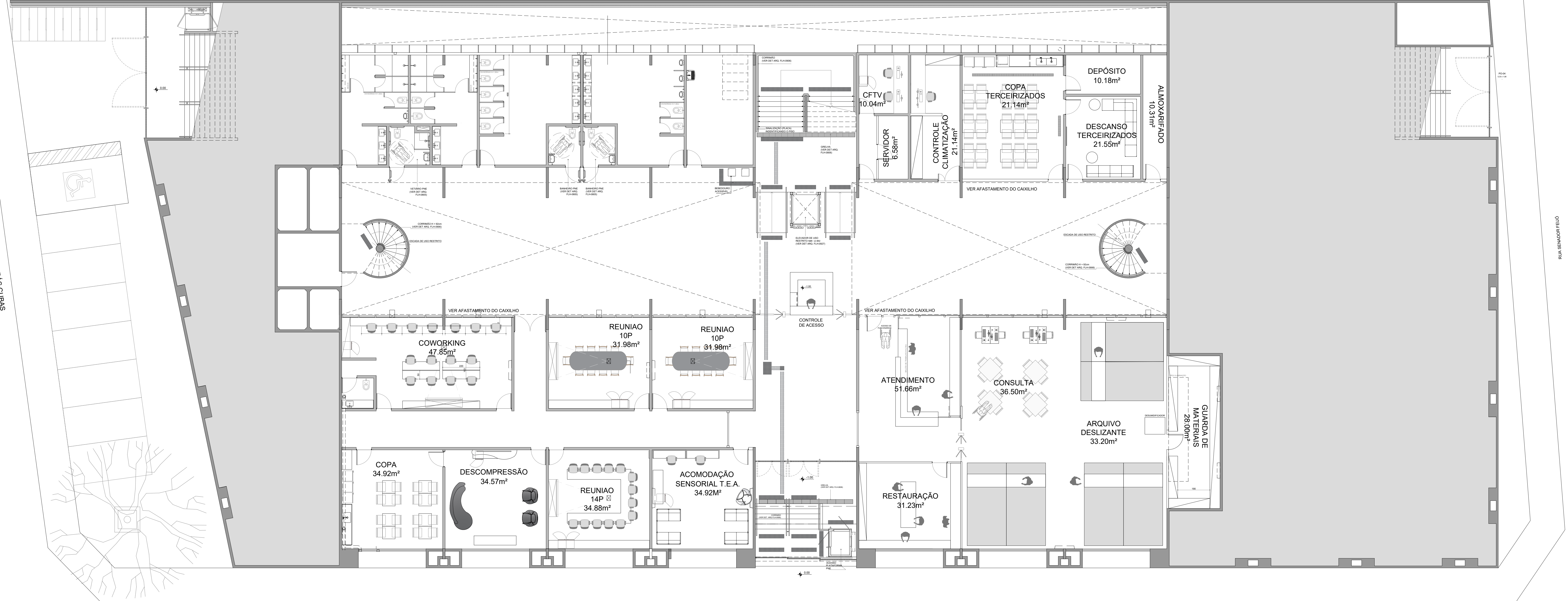
PAVIMENTO SUBSOLO
