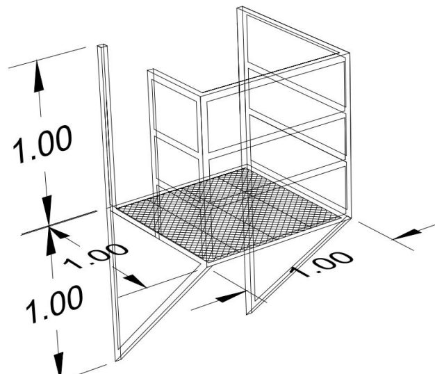
Vista em perspectiva da plataforma de serviços da caixa d'água medidas em metro
